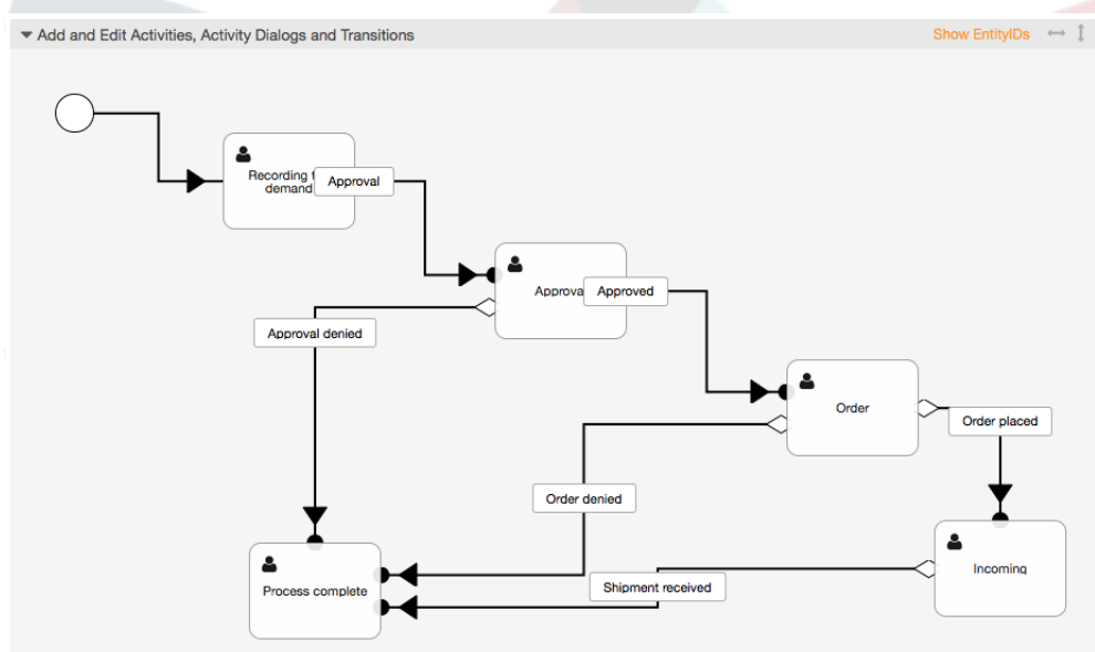
図: 本の注文の完全なプロセス・パス
