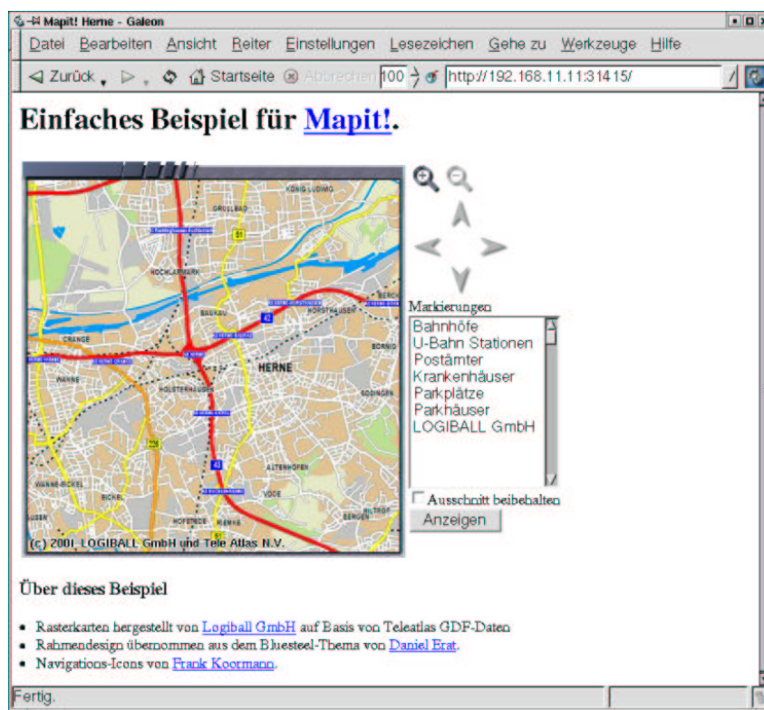
Abbildung 13.1.: Vom MapIt! Webserver generierte Seite mit präsentierter Karte „Herne“
